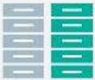
AI/ML
